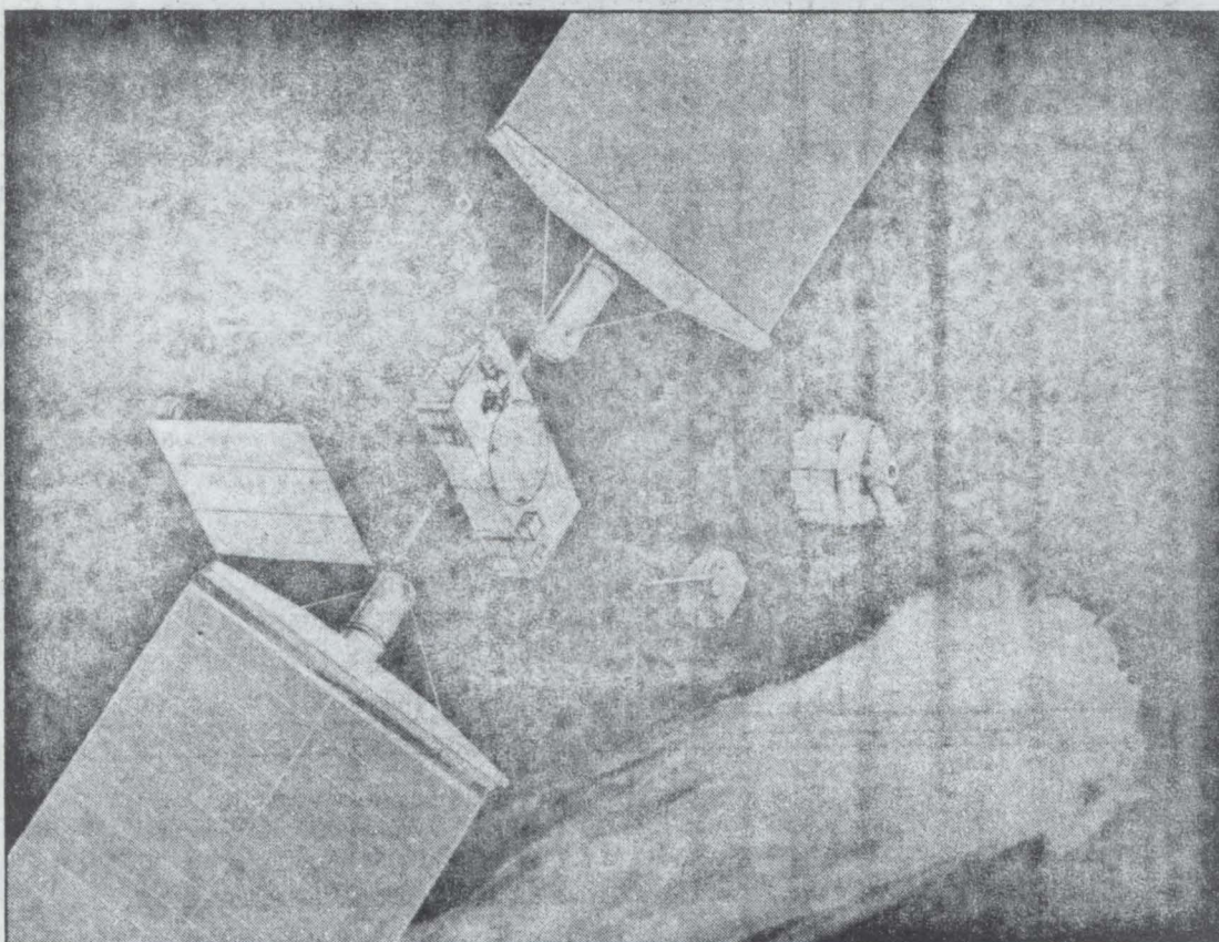
Jonraketen skjuter iväg ett instrumentpaket mot kometen. Kometen blir synlig från jorden 1985 och det planerade rymdmötet ska äga rum 1986.
